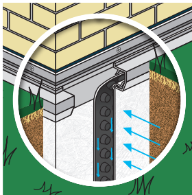
ND "Clic" Grundmauer Drain- und Schutzsystem mit ND 100
